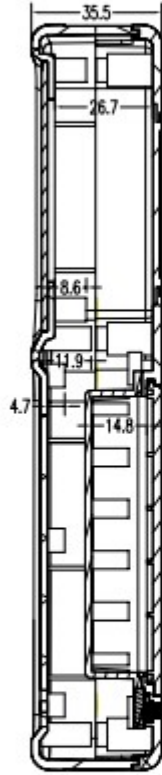
剖视图 A-A
